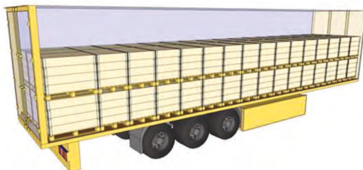
Figuur 12: Pallets stuwen in een voertuig met XL-code
