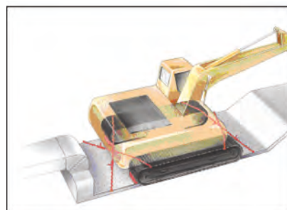
Figuur 37: Diagonaalsjorren
