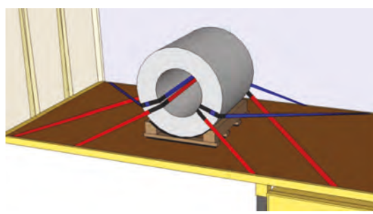
Figuur 65: Rol met gemiddeld gewicht
