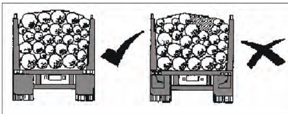
Figuur 50: Correct (links) en incorrect (rechts) geladen rondhout
