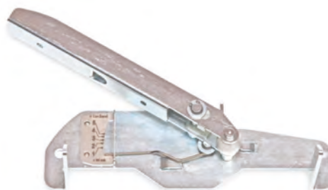
Figuur 23: Instrument voor het meten van de spankracht
