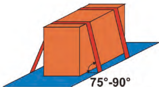
Figuur 41: Neersjorren
